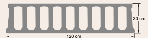
LOSA ALVEOLAR PERALTE 30
