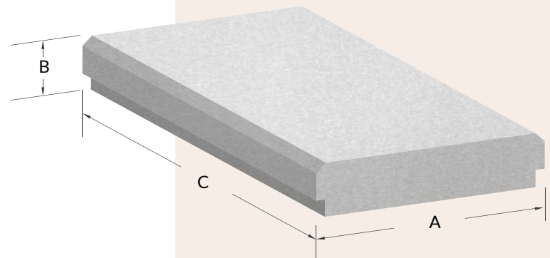
Bovedilla para Semiviguetas
